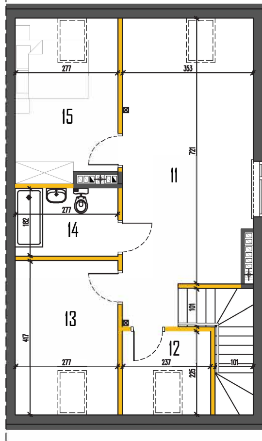
RZUT PODDASZA
