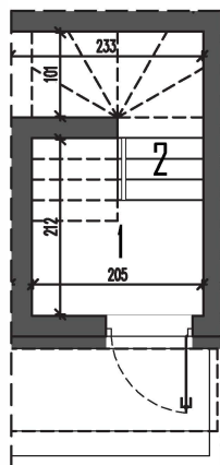
RZUT PARTERU
